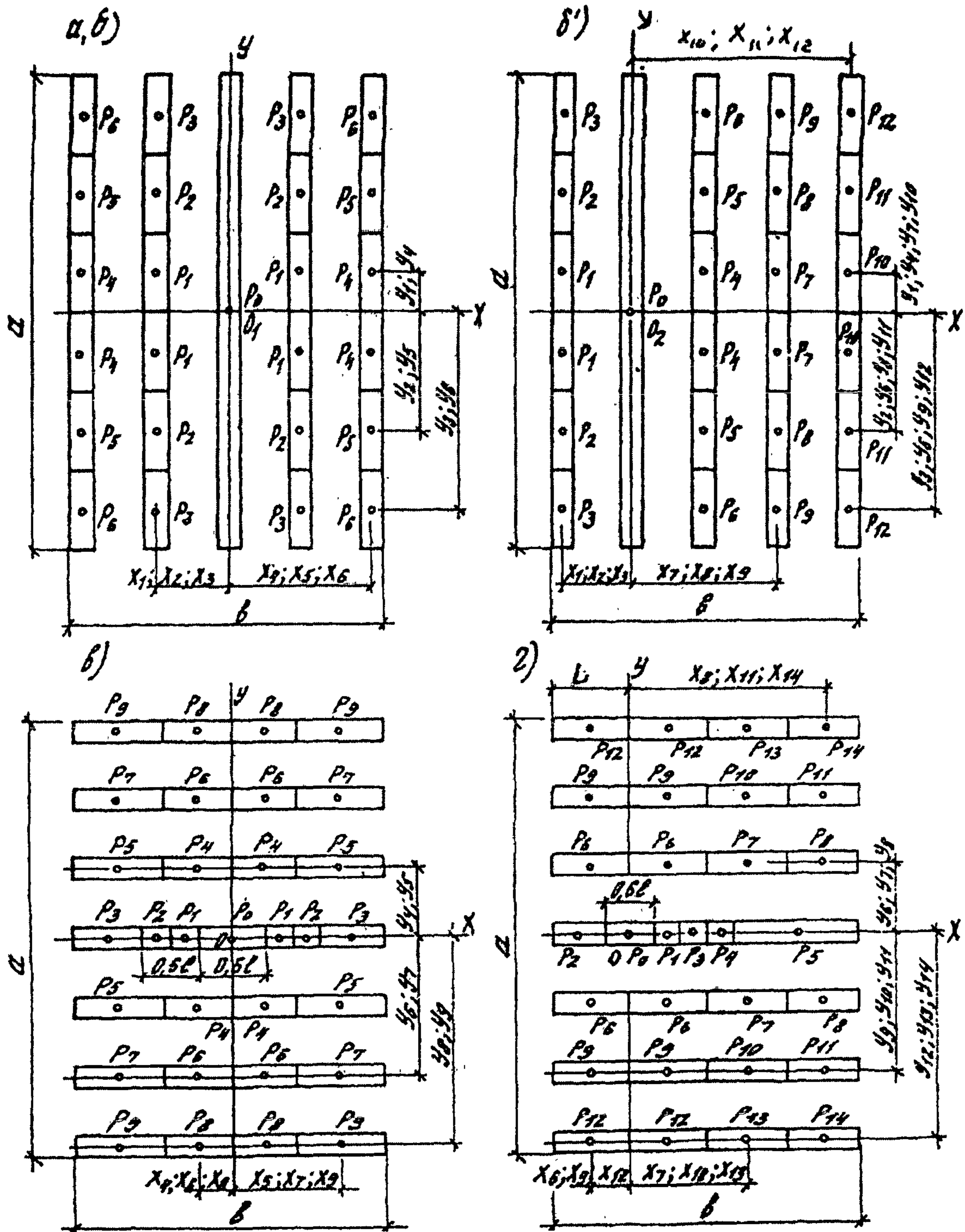
a, в – нагрузки, равномерно распределенные по длине параллельных следов (от прокладок под тяжелые предметы, от штабелей цилиндрических валов и др.) при b \leq 4,4l ; a > b ; б , б' , г – то же, при b > 4,4l ; a > b
